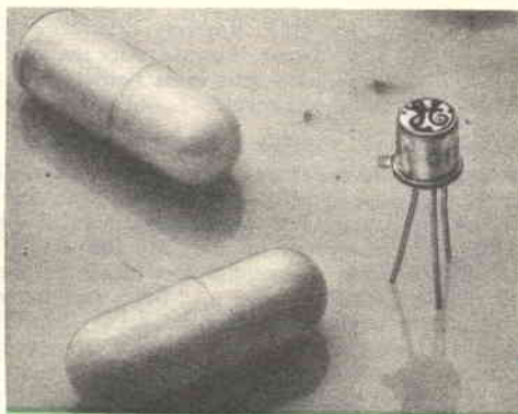
I diodi a tunnel rappresentati in fotografia e prodotti dalla General Electric stanno prendendo larga diffusione e sono usati in apparecchi prodotti in serie.
