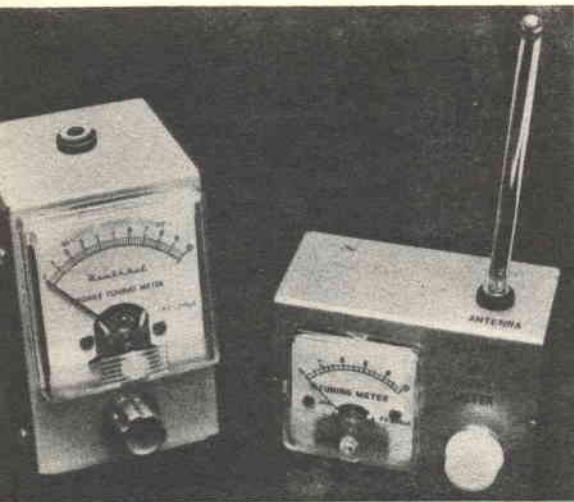
Questi due misuratori di intensità di campo, destinati al controllo di apparecchi portatili, hanno magneti fissati al pannello posteriore per fissarli al cruscotto dell'automobile.
