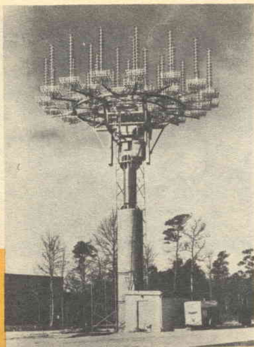
Questa nuova antenna a fascio a 33 elementi elicoidali è stata realizzata per seguire la corsa dei satelliti.
